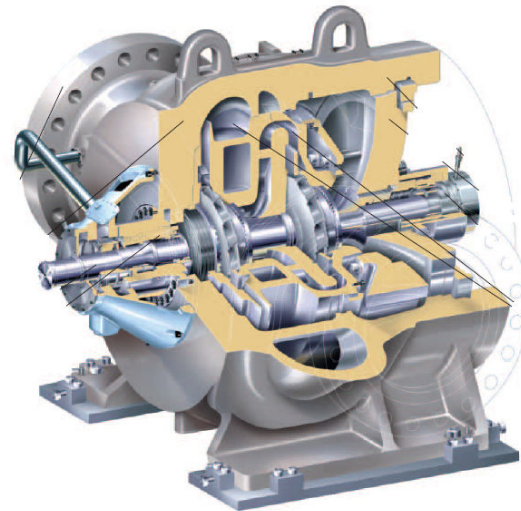
সেন্ট্রিফিউগাল কম্প্রেসর
