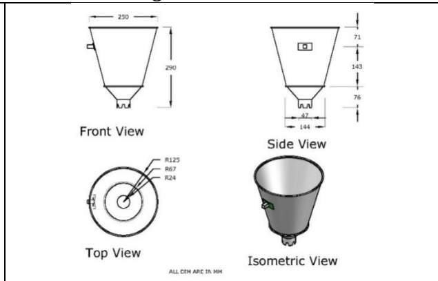
Fig. 41. Fertilizer chamber
