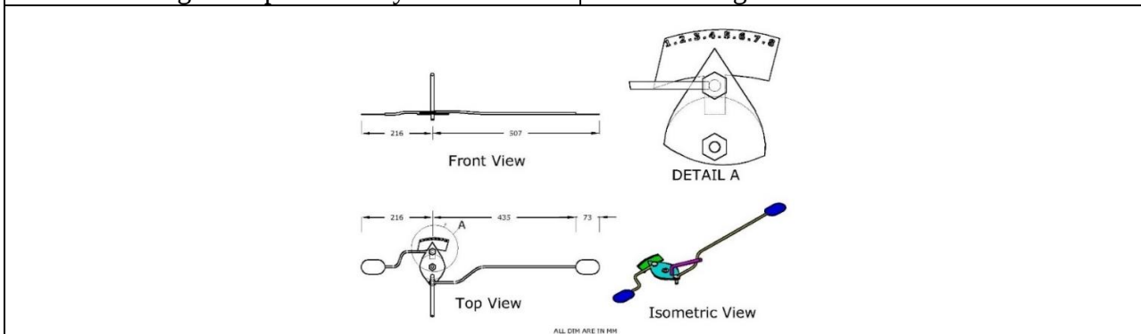
Fig. 42. Fertilizer control lever
