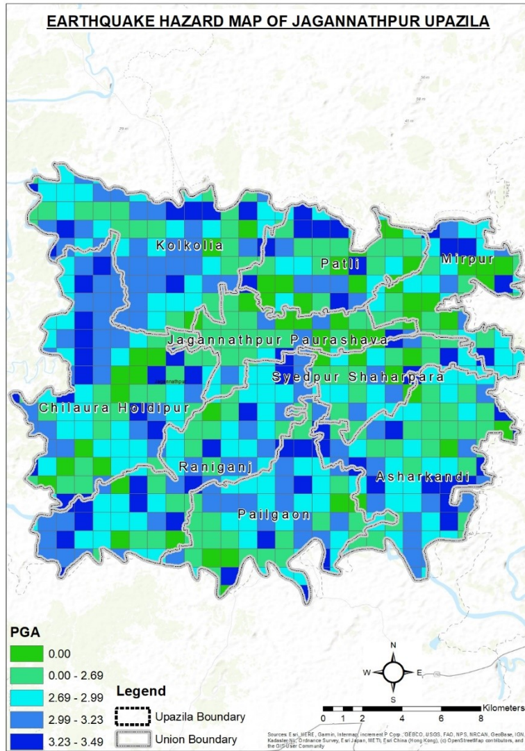
চিত্র ৩-২. জগন্নাথপুরের ভূমিকম্পের ঝুঁকির মানচিত্র
