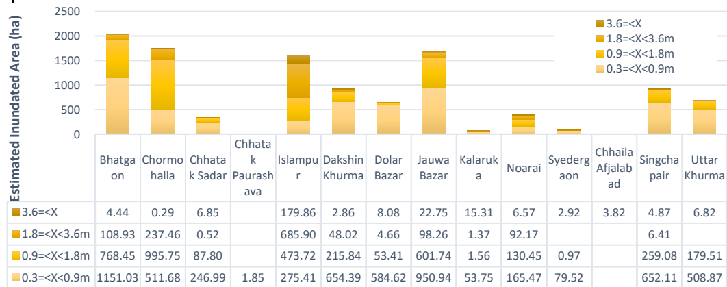
চিত্র ৪-২ BWDB এর পানির বিপদসীমায় পানির স্তর সহ ধানক্ষেতের প্লাবিত এলাকা
