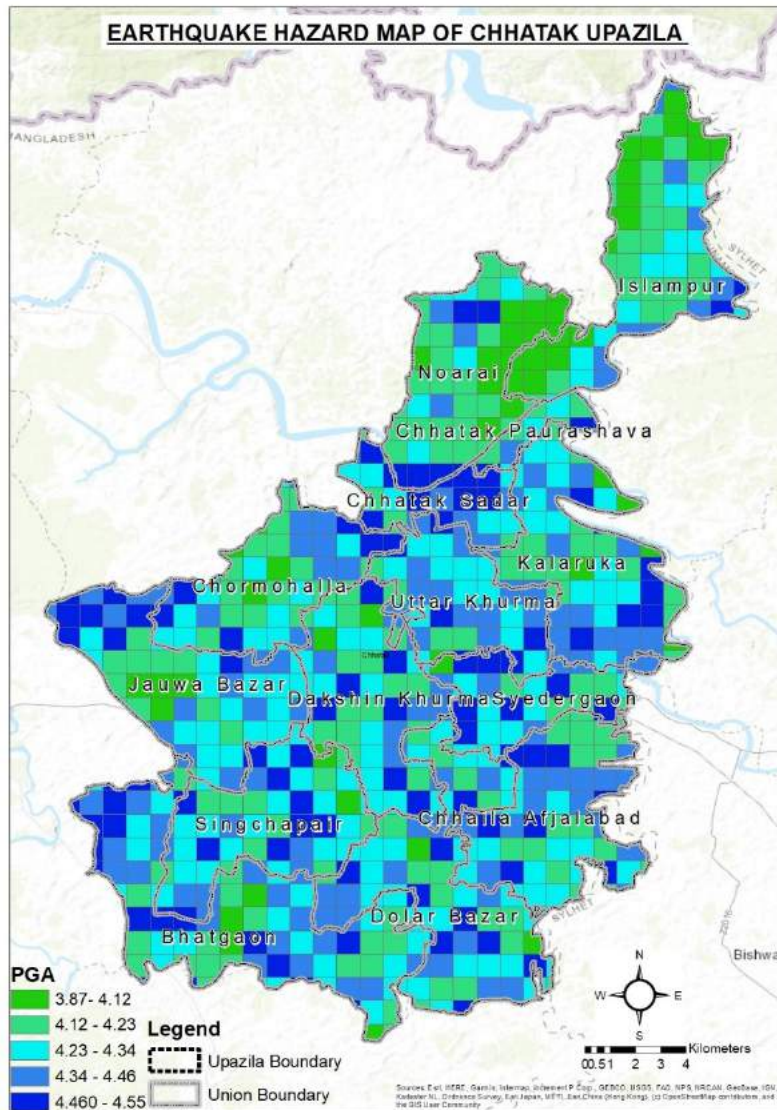
চিত্র ৩-২ ছাতকে ভূমিকম্পের ঝুঁকির মানচিত্র
