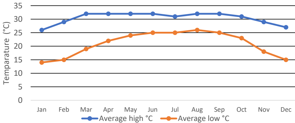
চিত্র ২-৫ গড় তাপমাত্রা
