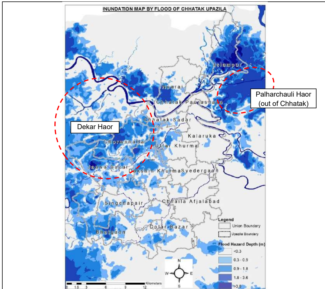
চিত্র ৩-১ ছাতক উপজেলায় নদীর বন্যা আপদের মানচিত্র
