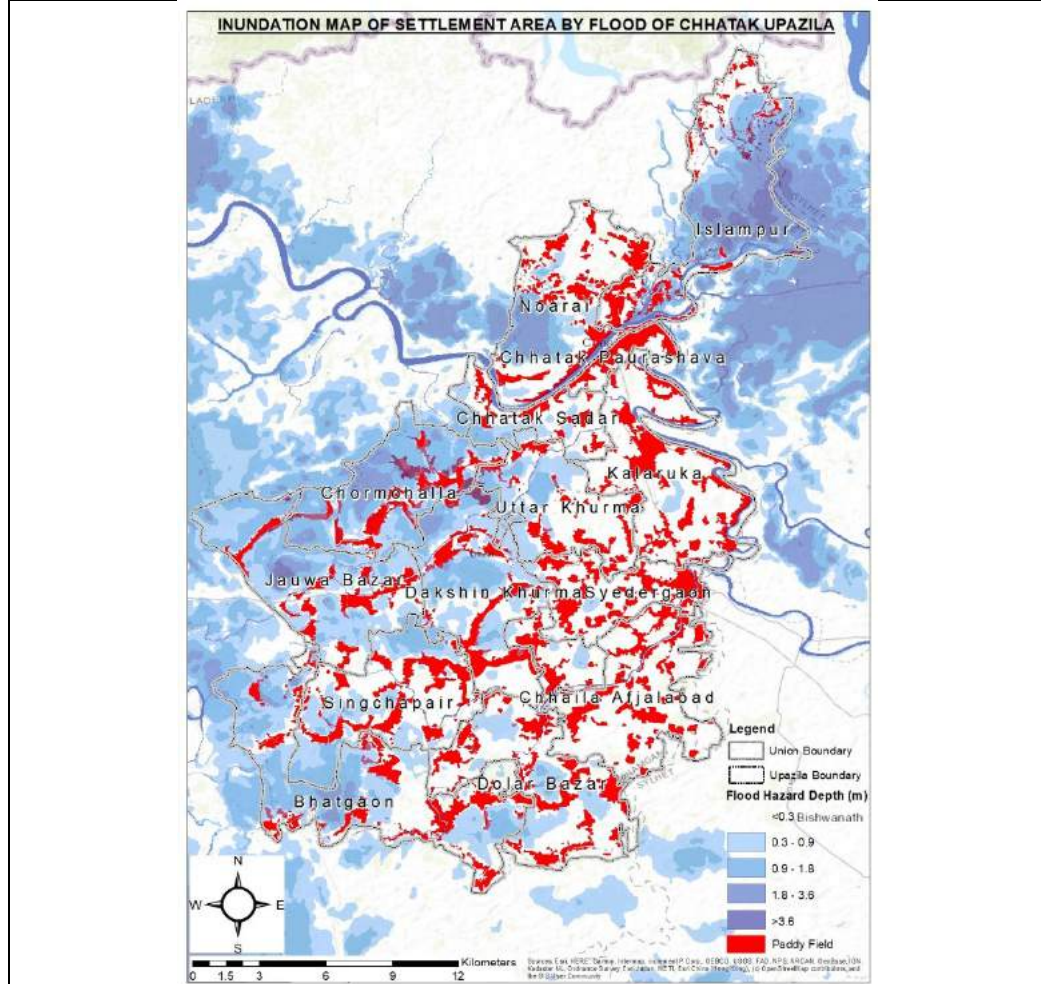
চিত্র ৪-৫ BWDB এর পানির বিপদসীমায় পানির স্তর সহ প্লাবিত এলাকা
