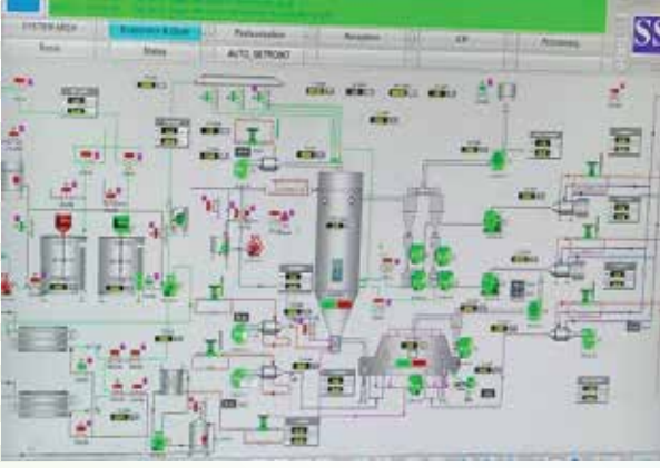
সিরাজগঞ্জের বাঘাবাড়িঘাটে গুড়োঁ দুধ উৎপাদন কারখানা এর প্রসেসিং লে আউট
