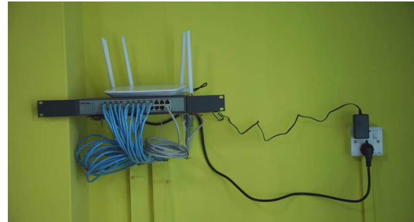
চিত্র ০৮ – রাউটার ও ল্যান সংযোগ
