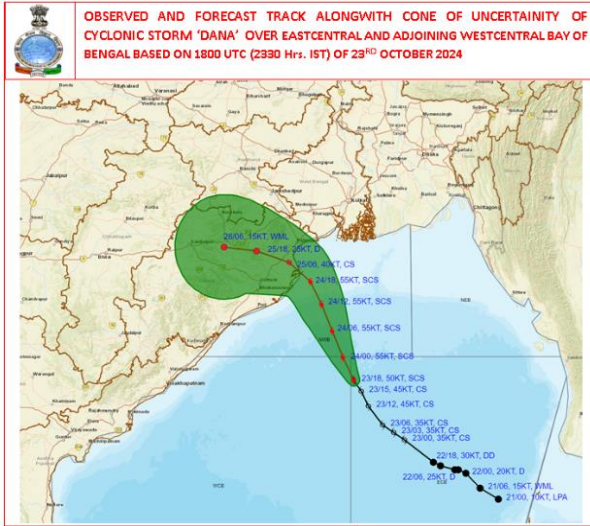
চিত্র-১: ঘূর্ণিঝড়ের সম্ভাব্য গতিপথ (লাল বৃত্ত) এবং পূর্ব অবস্থান (কালো বৃত্ত)
