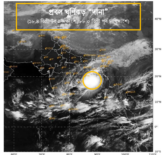
চিত্র-২: স্যাটেলাইট চিত্রে ঘূর্ণিঝড়টির অবস্থান (২৪-১০-২০২৪ খ্রি. সকাল ০৮.১৫ টা)
