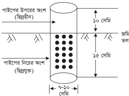
চিত্র ১৪। এডব্লিউডি পাইপ তৈরি এবং স্থাপন পদ্ধতি।
